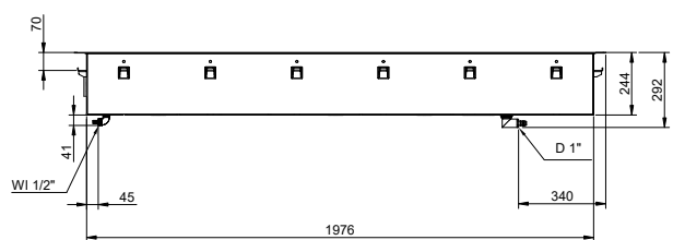
Zadní strana
